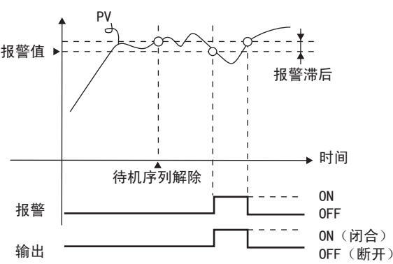
报警类型：偏差下限待机序列 ON
