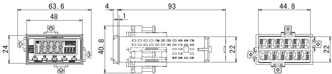
无螺钉夹具端子台型
